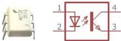
Fig. 6 - OPTOCOUPLER
